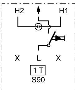
1T-vipupainike Erillinen lamppupiiri 2 lisäliitintä
