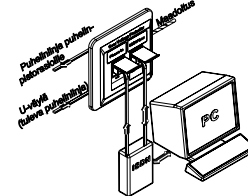
ISDN-ylijännitesuoja OP22
