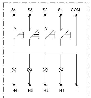
Pienjännitepainike PI4
