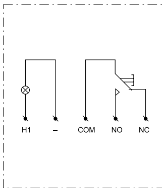
Pienjännitepainike PI1
