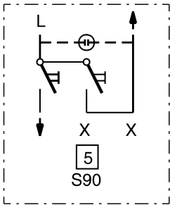
5-kytkin (sarja) 2 lisäliitintä
