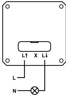
2-johdinkytkentä (SP300)
