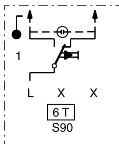
6T-vipupainike (Huom. avautuva/sulkeutuva, jousen paikka muutettavissa) 2 lisäliitintä
