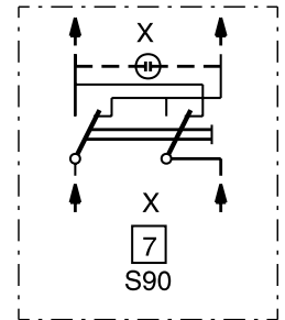
7-kytkin 2 lisäliitintä
