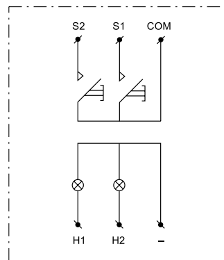
Pienjännitepainike PI2
