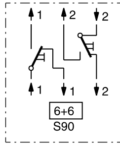
6+6-kytkin (vaihto/vaihto)
