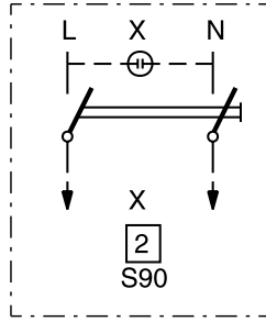
2-napainen 2 lisäliitintä
