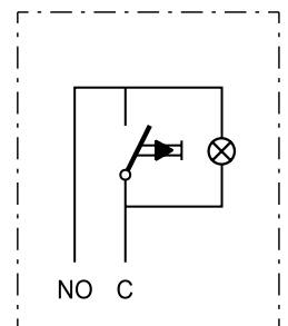
P5-painike ruuviliittimin
