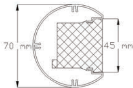
MCR70 pylväs runko EL 14 120 55 VA 14 120 05
