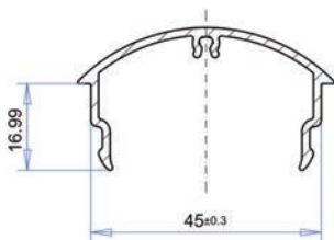
MCR70 kansi pyöreä EL 14 120 56 VA 14 120 06
