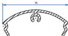
MCR50 kansi pyöreä EL 14 661 03 VA 14 661 06
