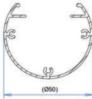
MCR50 pylväs runko EL 14 661 02 VA 14 661 05
