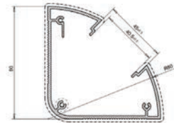
TRI80 pylväs runko EL 14 122 46 VA 14 122 45
