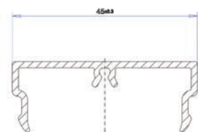
MC1 kansi suora EL 14 111 12 VA 14 111 02
