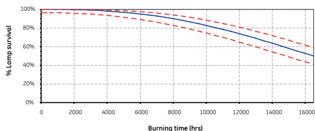
Lamp survival CMH MR16 Ultra 35W EM
