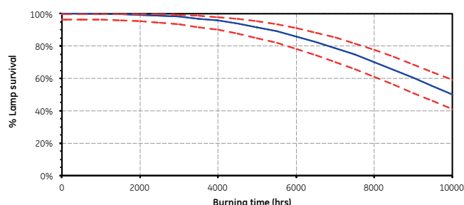
Lamp survival CMH MR16 Ultra 35W EM
